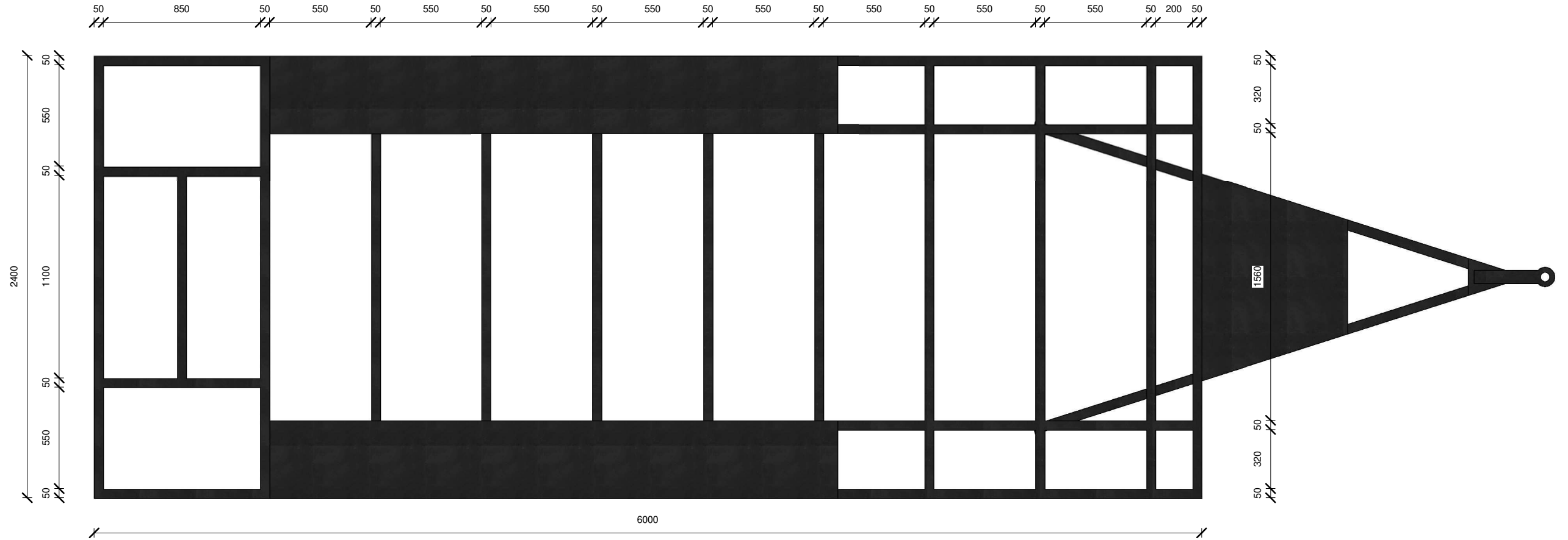
1 TRAILER PLAN 1 : 25
